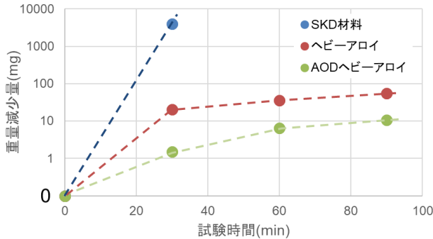
Fig. アルミ溶湯を用いた溶損試験結果
