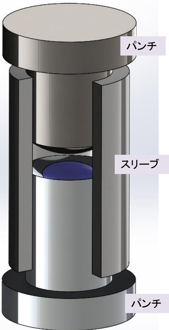
Fig. レンズ成形の模式図
