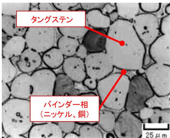
Fig. 「ヘビーアロイHAC2」の内部組織写真
