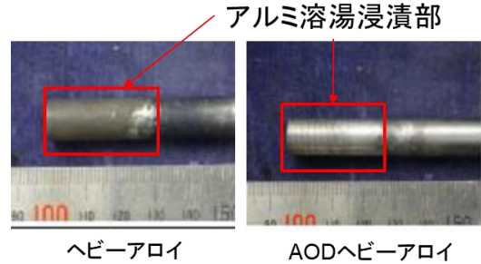
Fig. 90min浸漬後の試験片外観写真
