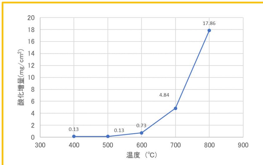
Fig. 2 HAF1 温度と酸化増量の関係
