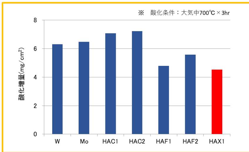
Fig. 1 各材料の酸化増量比較
